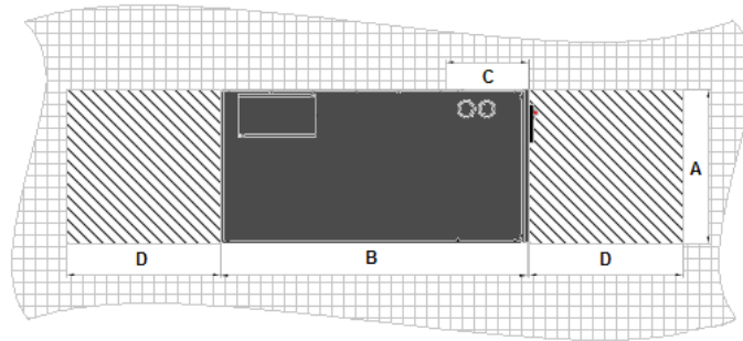
Требуемое пространство для Серии B
